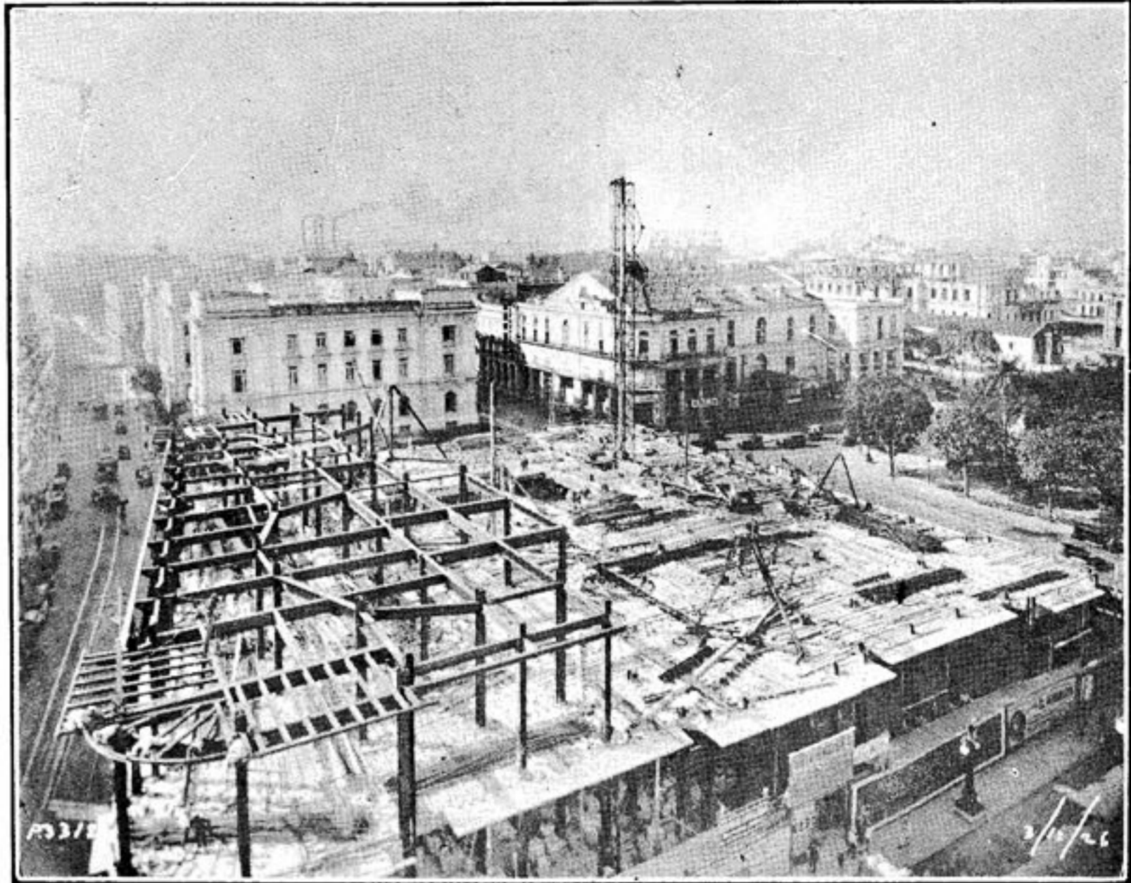
Perspectiva de la construcción del formidable esqueleto de hierro, obra maestra de la "American Steel Company of Cuba".
