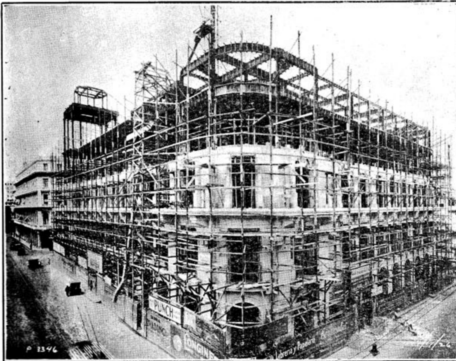
Otra perspectiva, en la que la sólida piedra de Capellania, de la Casa Almo Strenta, avanza, en orgullosa competencia con el herraje, hacia el término de la construcción.
