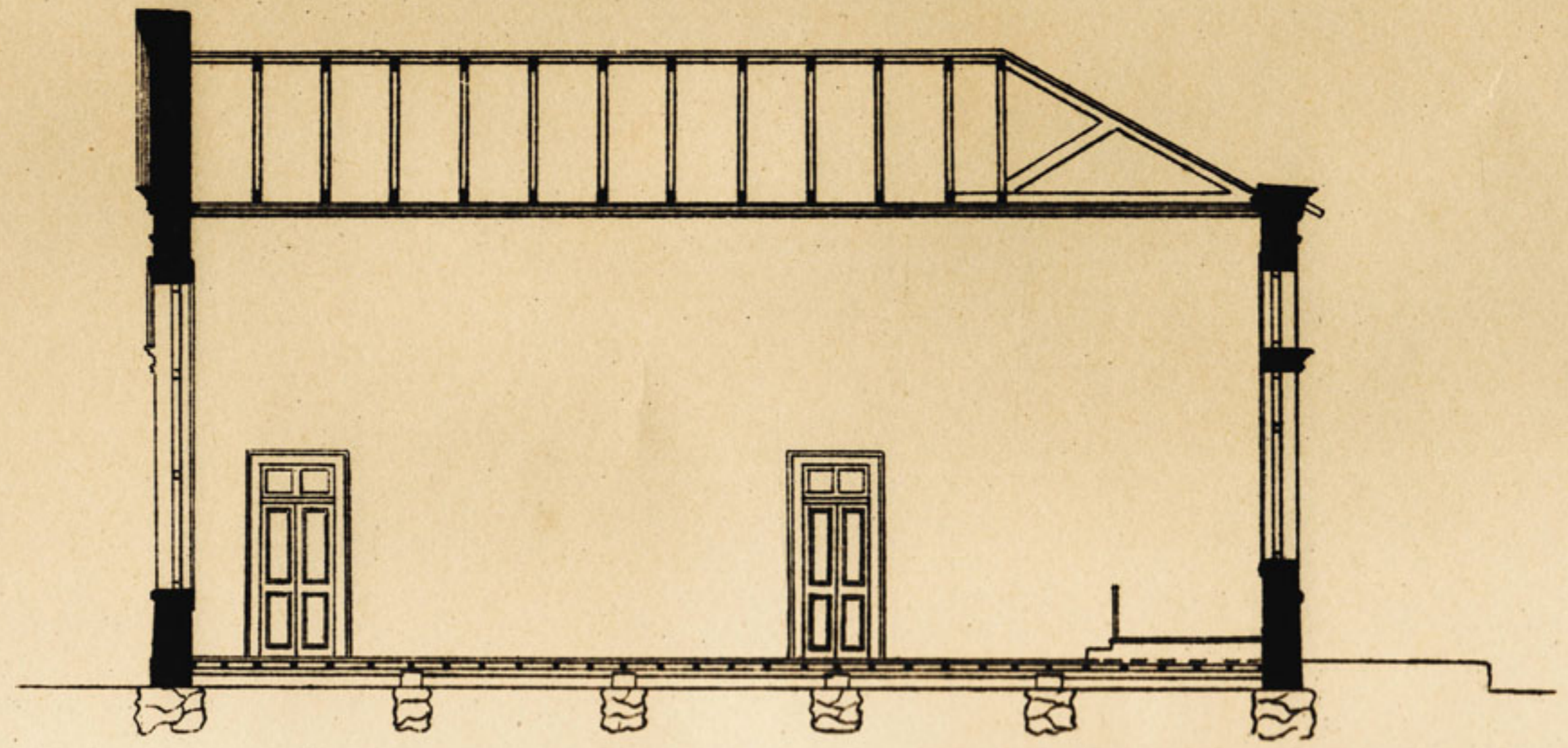
Corte de una de las salas de clases
